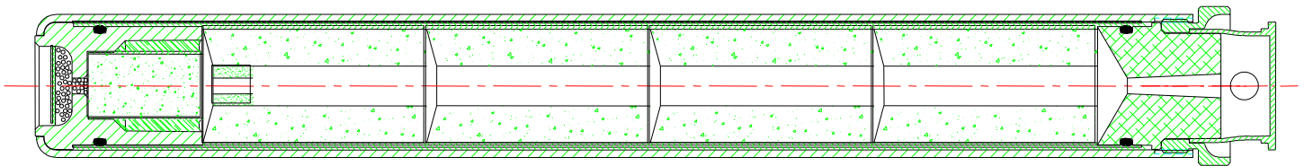
Moteur Pro29-4G assemblé (sans allumeur)
